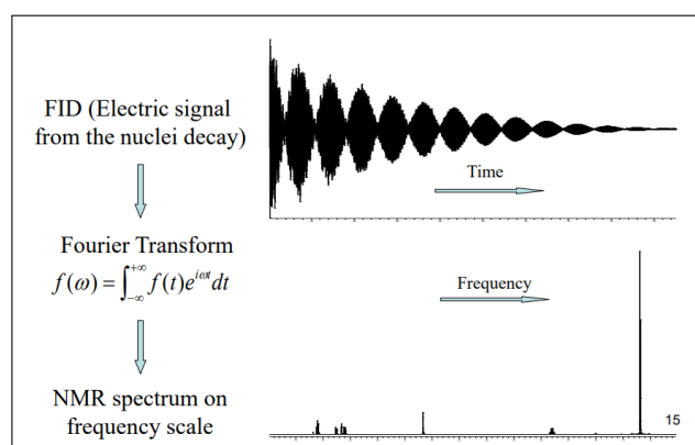
Figura 20: Algoritmo di gestione di uno FT-NMR
