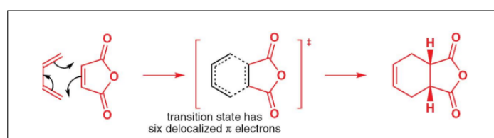
Figura 11: Reazione di Diels-Alder con TS mostrato
