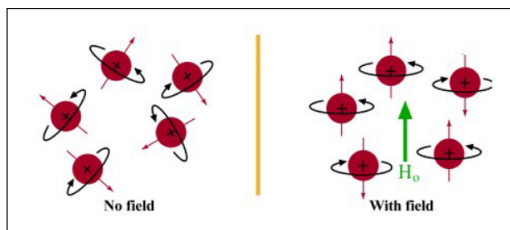
Figura 18: Disposizione dei nuclei degli atomi in presenza e assenza di un campo magnetico
